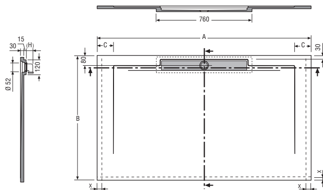
LineY rectangulaire / Smooth / Slate
