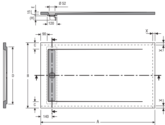
LineX rectangulaire / Smooth / Slate
